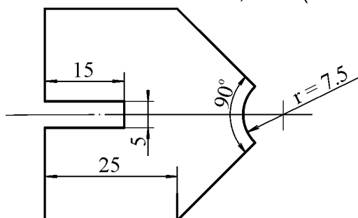
ŠABLONA PRO POLOMĚR ŠPIČKY, HÁČEK A OZNAČENÍ
